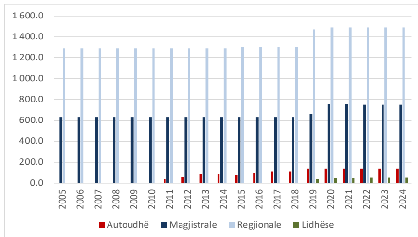
FIG. 16.2: RRUGË TË ASFALTUARA DHE TË PA ASFALTUARA 2005-2024
